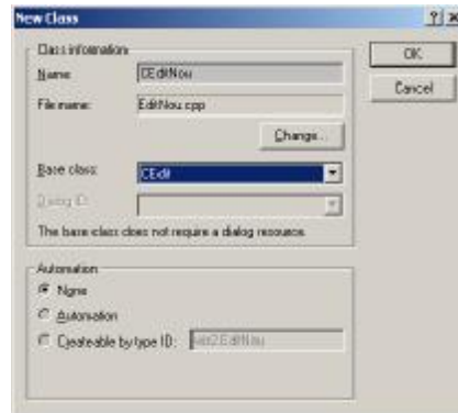
Figura 5.14 Definin noua clasă
