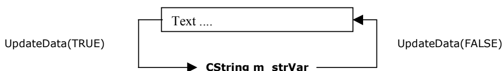
Figura 5.11 Transferul valorii între control și variabila mapată
