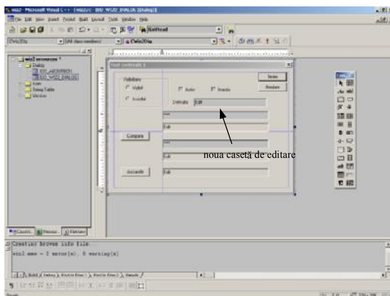
Figura 5.13 Casetă de editare de clasă derivată
