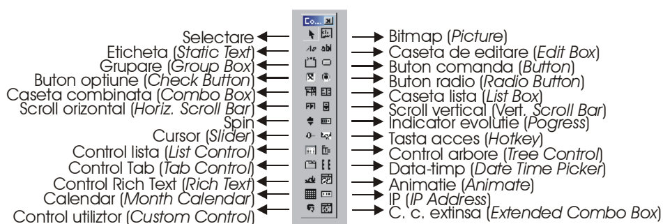
Figura 5.1 Controale disponibile
