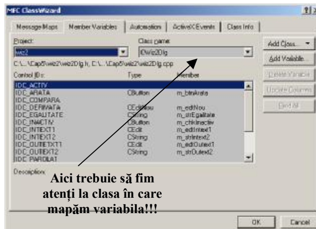
Figura 5.8 Maparea variabilelor
