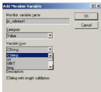
Figura 5.10 Variabilă Value
